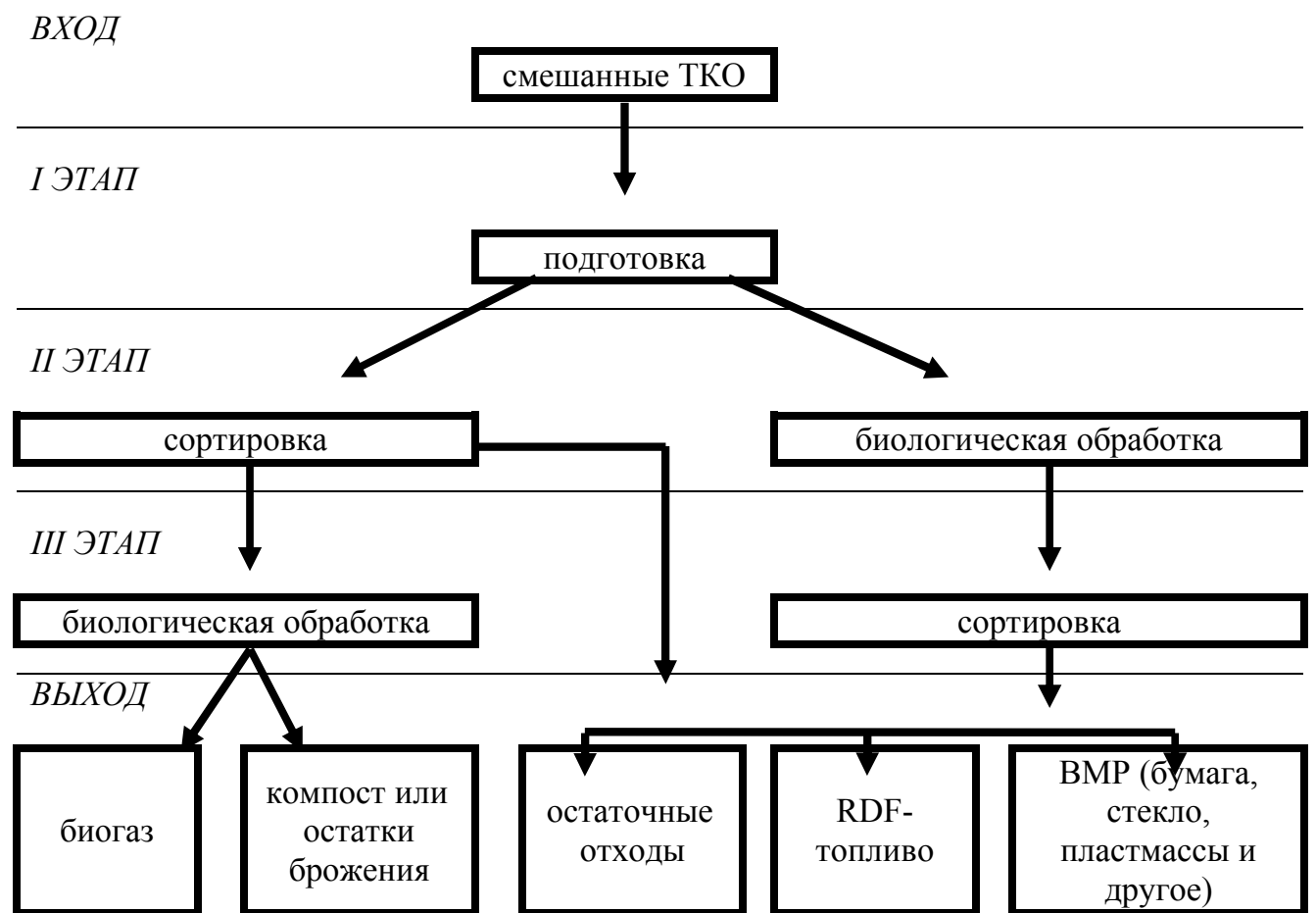
Рисунок. Способы механико-биологической обработки смешанных ТКО
